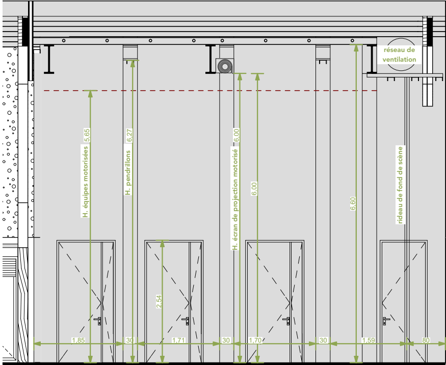
ZOOM Élévation (B)
