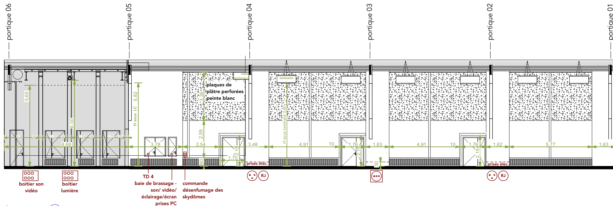
Élévation A
