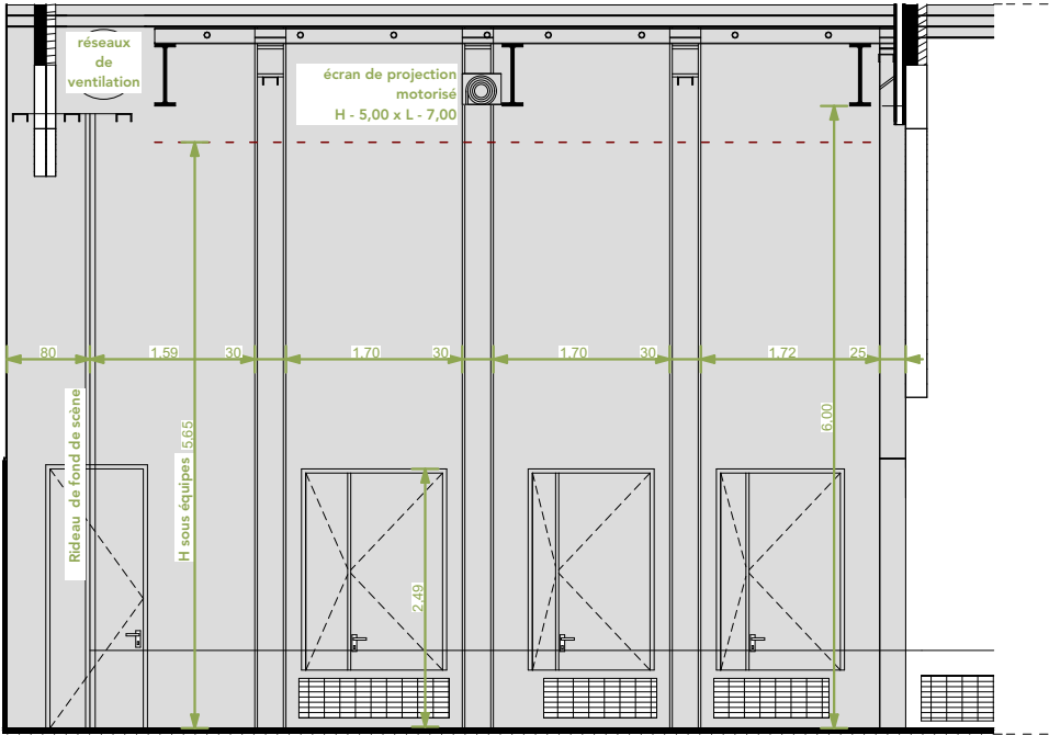
ZOOM Élévation (A)
