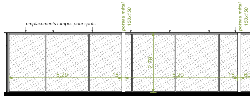
Élévation C
