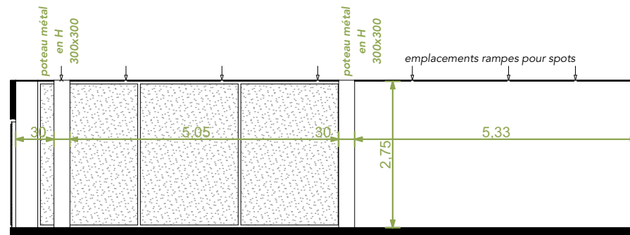
Élévation D
